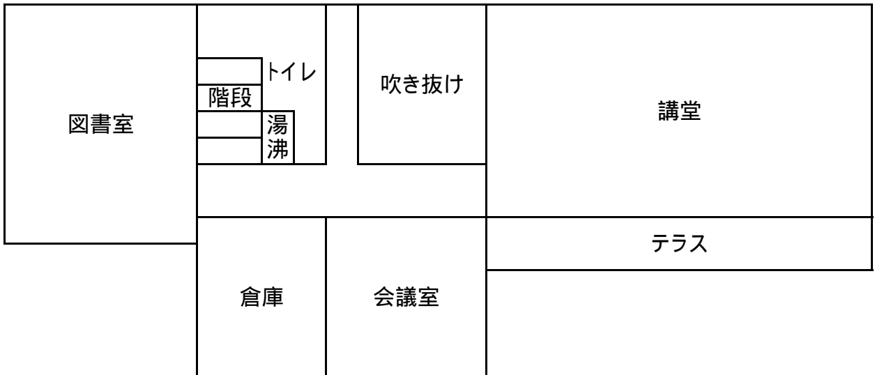
2階平面図
