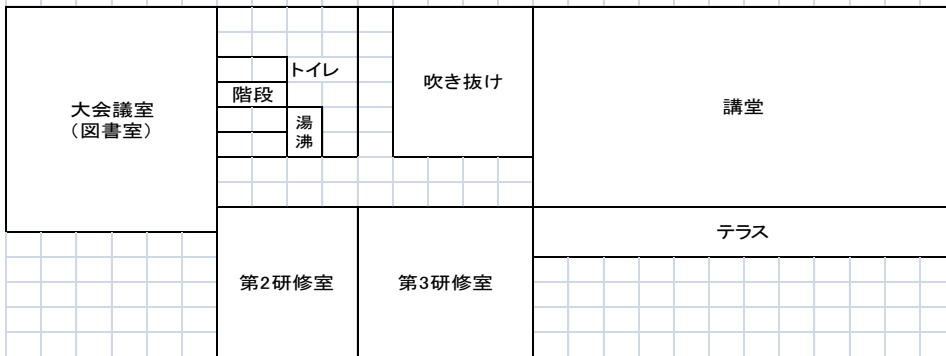
◆ 2階平面図 ◆
