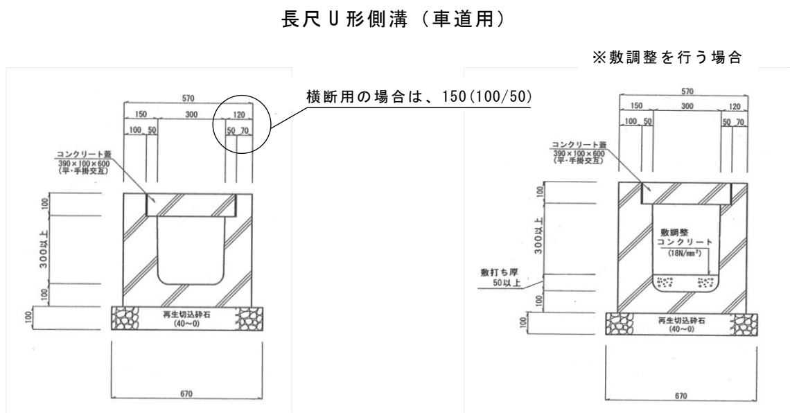
【図 2】道路側溝標準図
