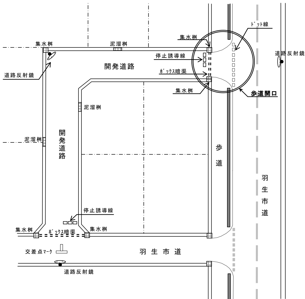
【図 9】＜参考＞道路築造標準図
